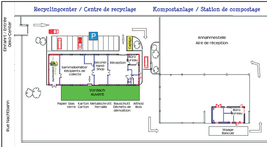
Übersichtsplan OEKO-CENTER Hesper Plan de l'OEKO-CENTER Hesper
